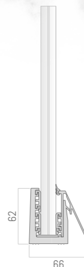
NINFA 50 MONTAGGIO SOPRA I MURETTI
