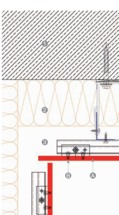
ANGLE RENTRANT
