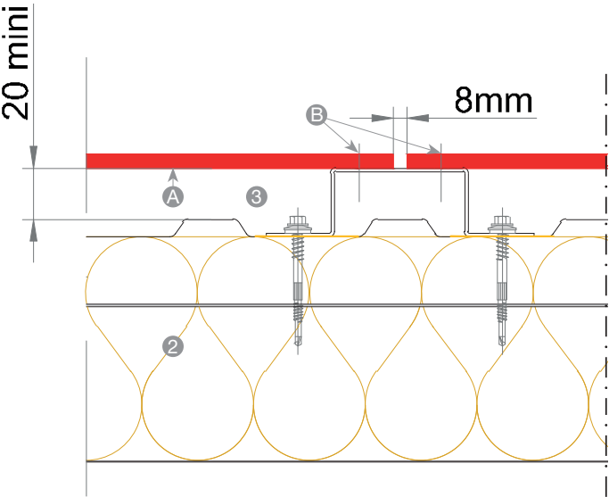
SECTION COURANTE
