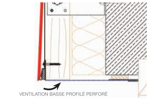
DÉTAIL LINTEAU
