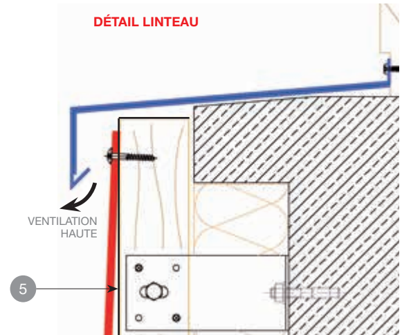
DÉTAIL APPUI DE FENÊTRE
