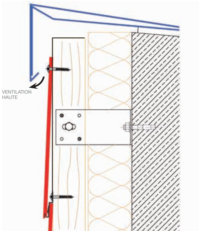
DÉTAIL COUVERTINE
