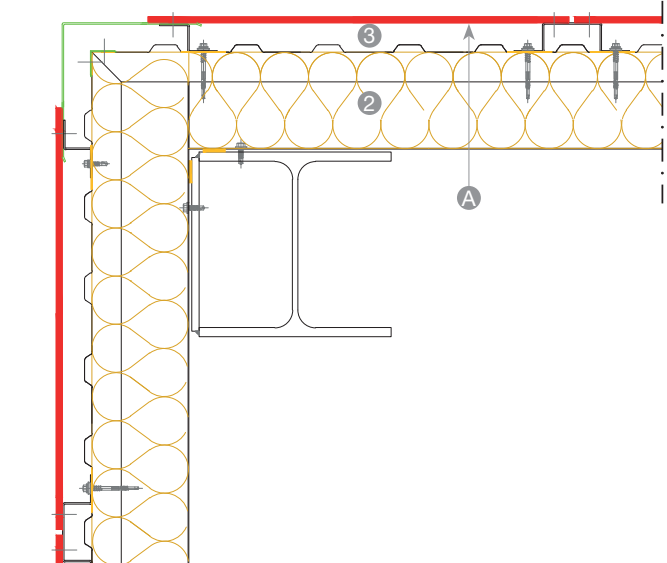
DÉTAILS D'ANGLE
