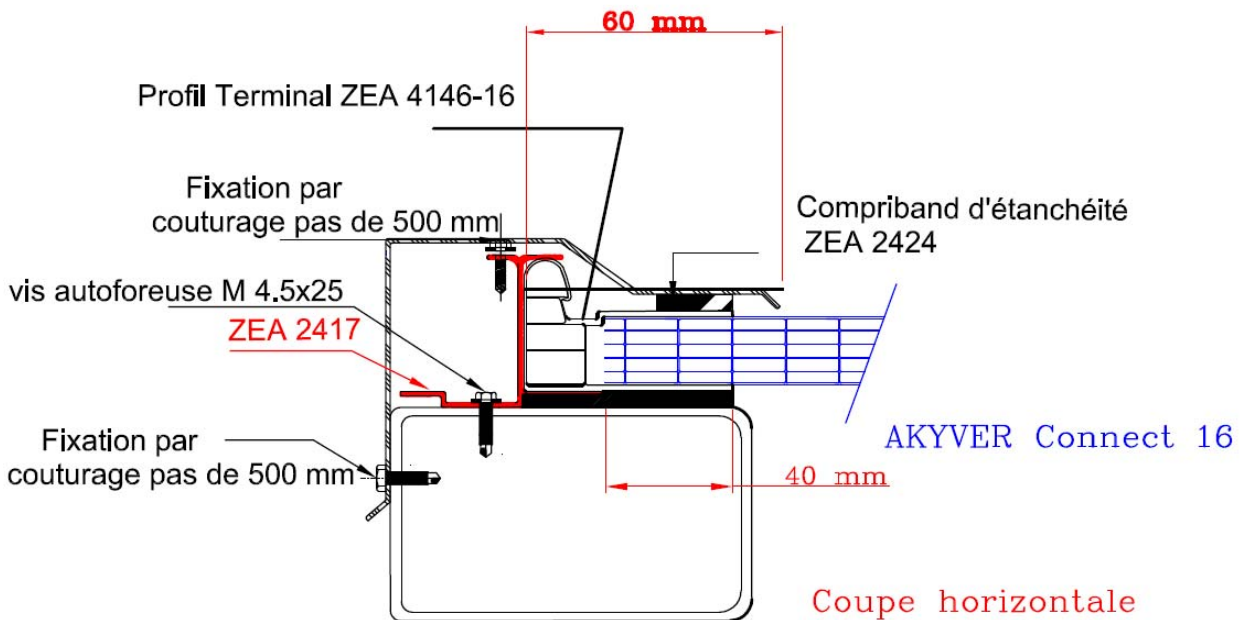
Figure 19c – Traitement extrémité avec profil terminal (uniquement dans le cas de bâtiments ouverts)
