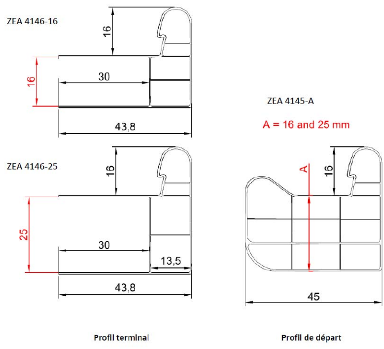
Figure 19a – Profil terminal, uniquement en bâtiment ouvert, et profil de départ
