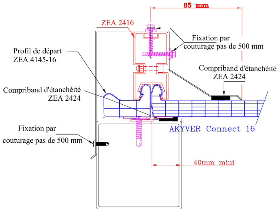
Figure 19b – Traitement extrémité avec profil de départ
