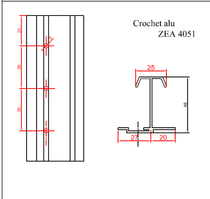
Figure 6 – Crochets de dépression en aluminium réf. ZEA 4000, ZEA 4000 renforcé, ZEA 4051 et ZEA 4028
