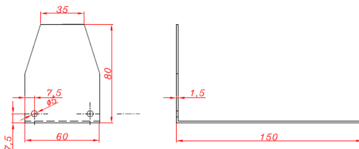
Équerre de retenue ZEA 3819 pour ZEA 2416
