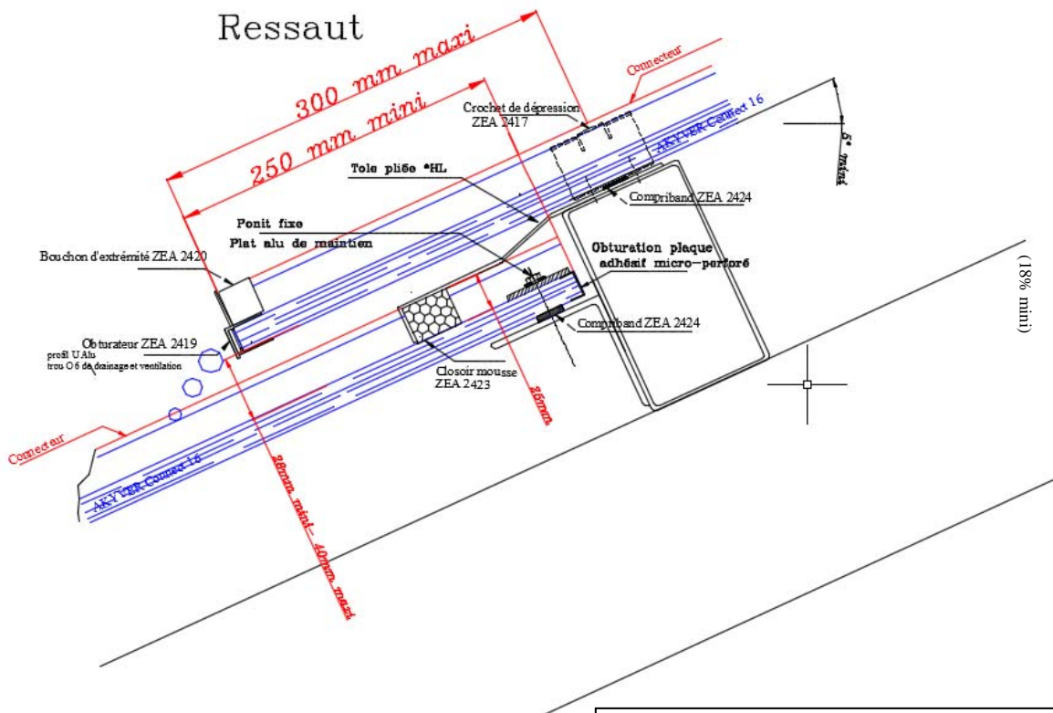
Figure 20 – Ressaut (plaques avec point fixe en tête, pente \geq 18\% )
