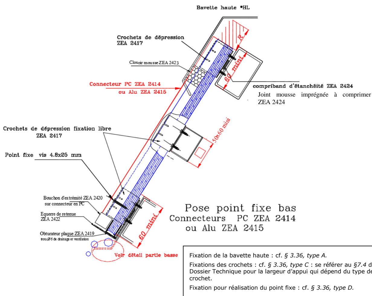
Figure 12 - Pose avec point fixe bas
