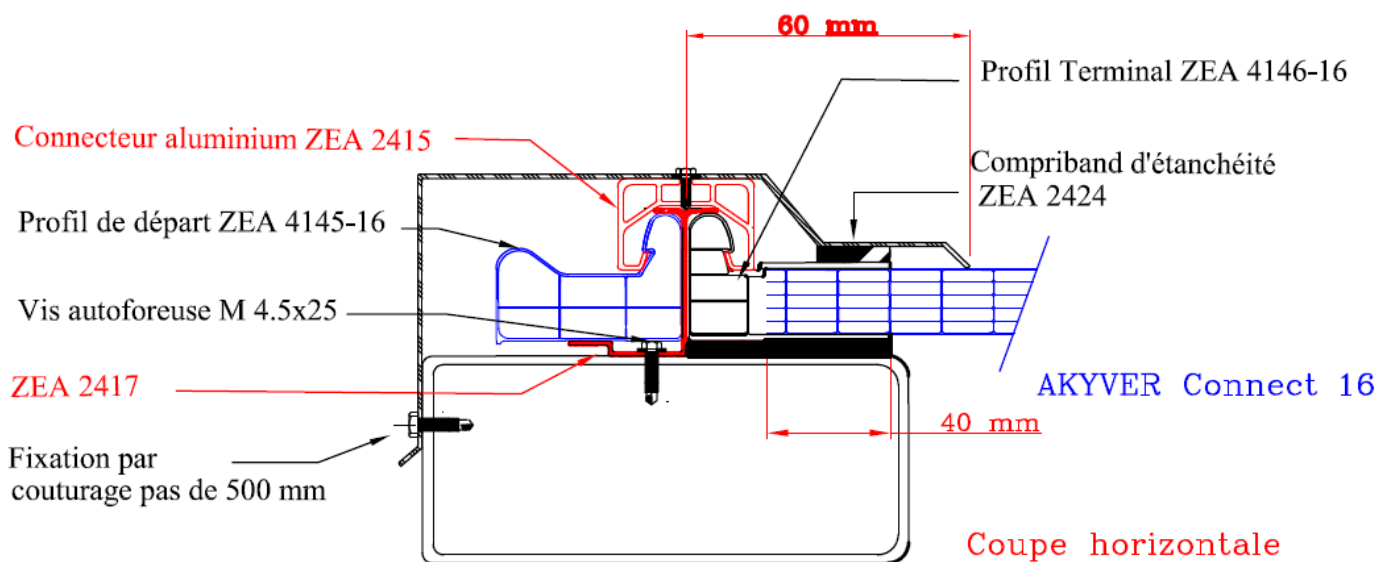
Figure 19d – Traitement extrémité avec association d'un profil terminal et de départ (uniquement dans le cas de bâtiments ouverts)
