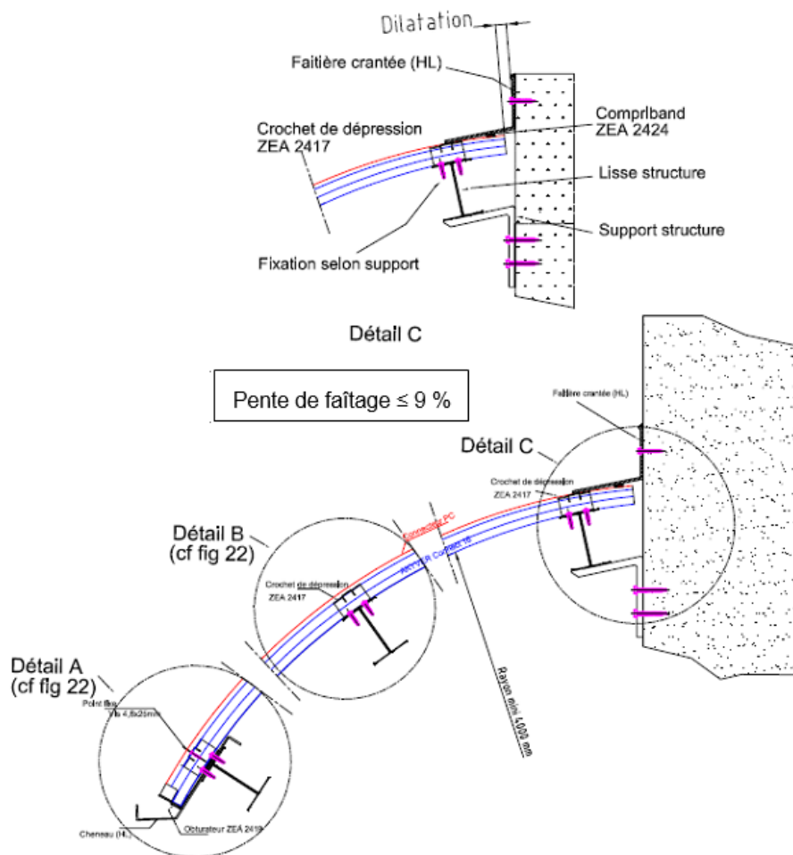
Figure 22 – Pose cintrée – Coupe longitudinale et transversale
