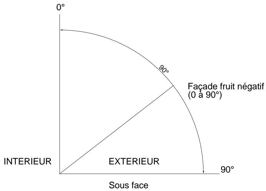
Figure 15 - Fruit négatif
