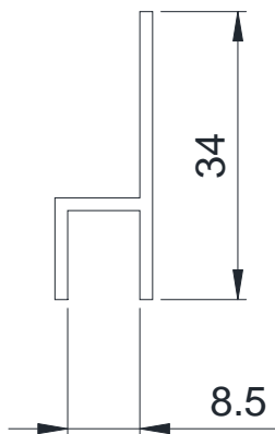
Figure 19bis – Profilé « chaise » pour fermeture des joints horizontaux
