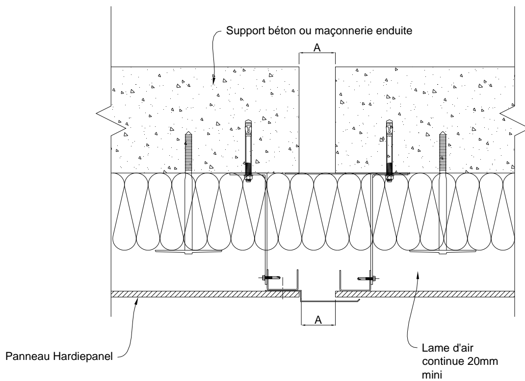
Figure B2 – Joint de dilatation de 12 à 15 cm
