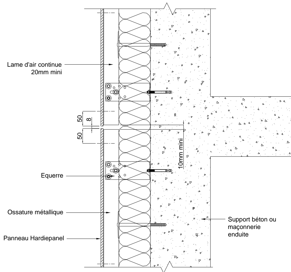
Figure B1 – Fractionnement de l'ossature au droit de chaque plancher
