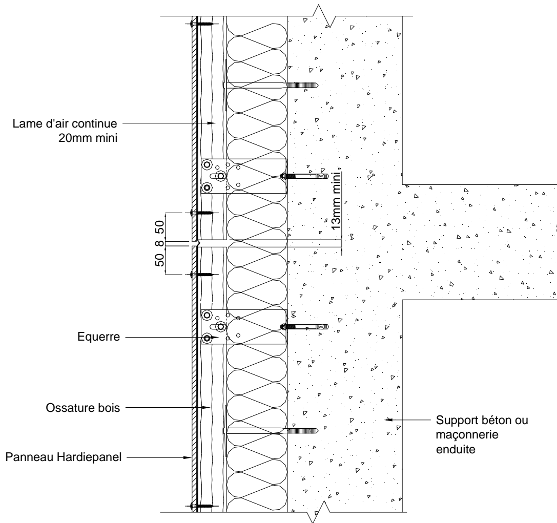
Figure A1 – Fractionnement de l'ossature au droit de chaque plancher
