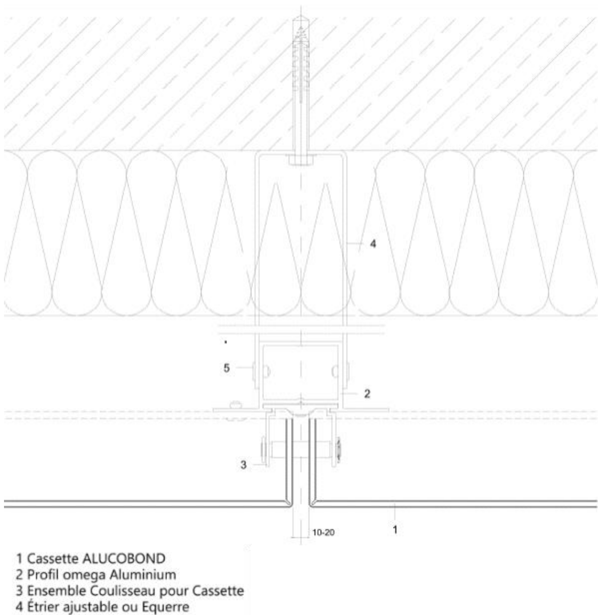
Figure 17 – Joint vertical entre cassettes – Système d'ossature POE1 avec coulisseau et équerres en quinconce – Pose sur maçonnerie (Coupe horizontale)
