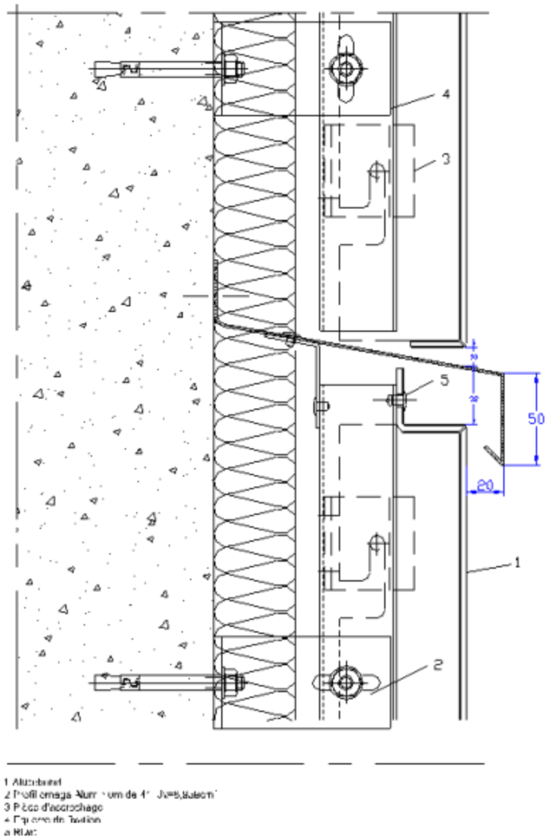
Figure 27 – Fractionnement de la lame d'air (Coupe verticale) (Système POB1)
