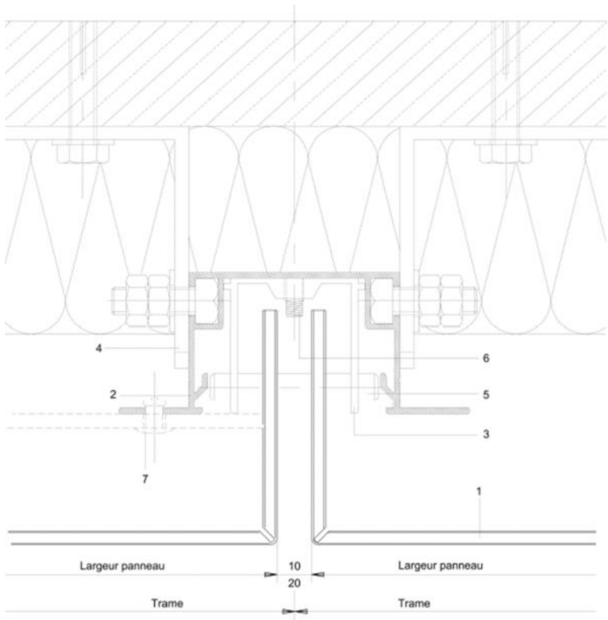
Figure 16 – Joint vertical entre cassettes – Système d'ossature POB1 avec coulisseau et équerres en quinconce – Pose sur maçonnerie (Coupe horizontale)
