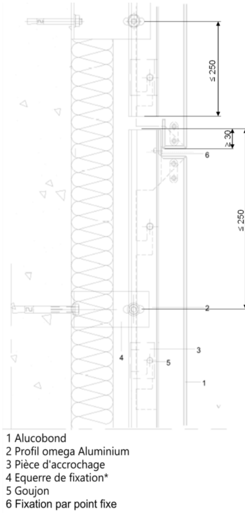
Figure 29 – Fractionnement de l'ossature (Système POB1)
