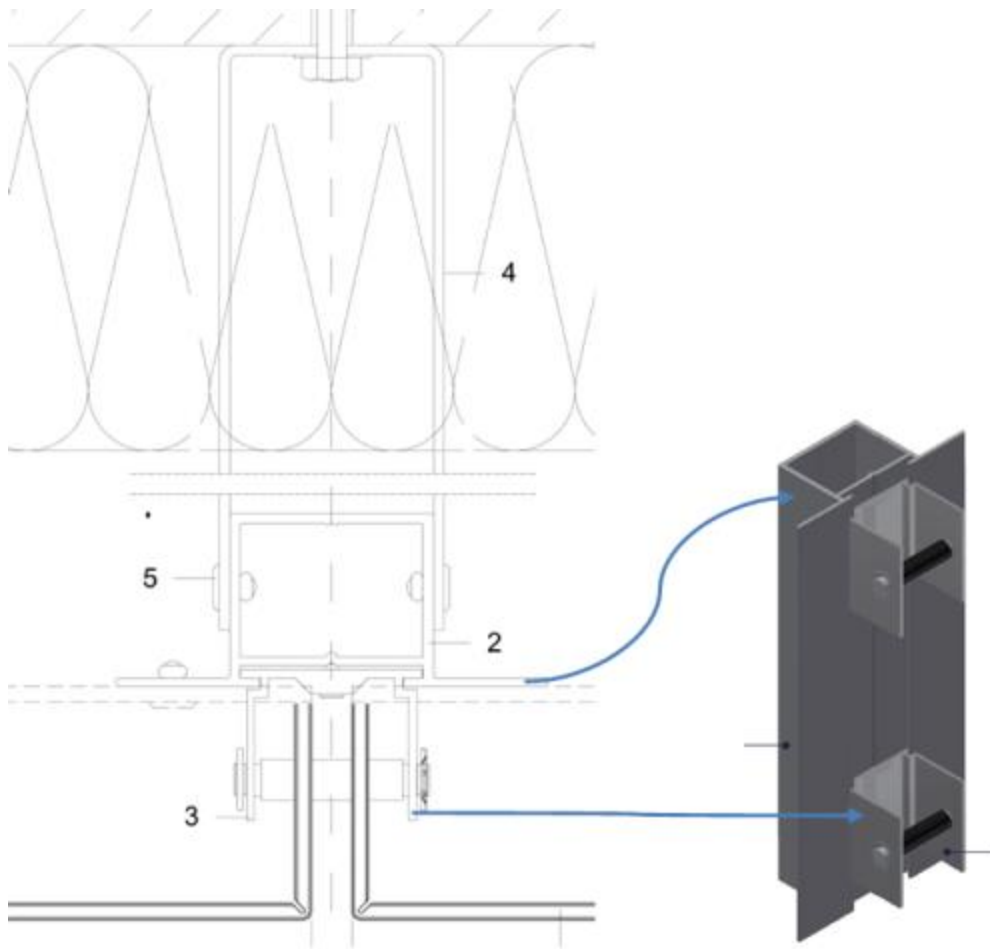
Figure 13 –Système POE1
