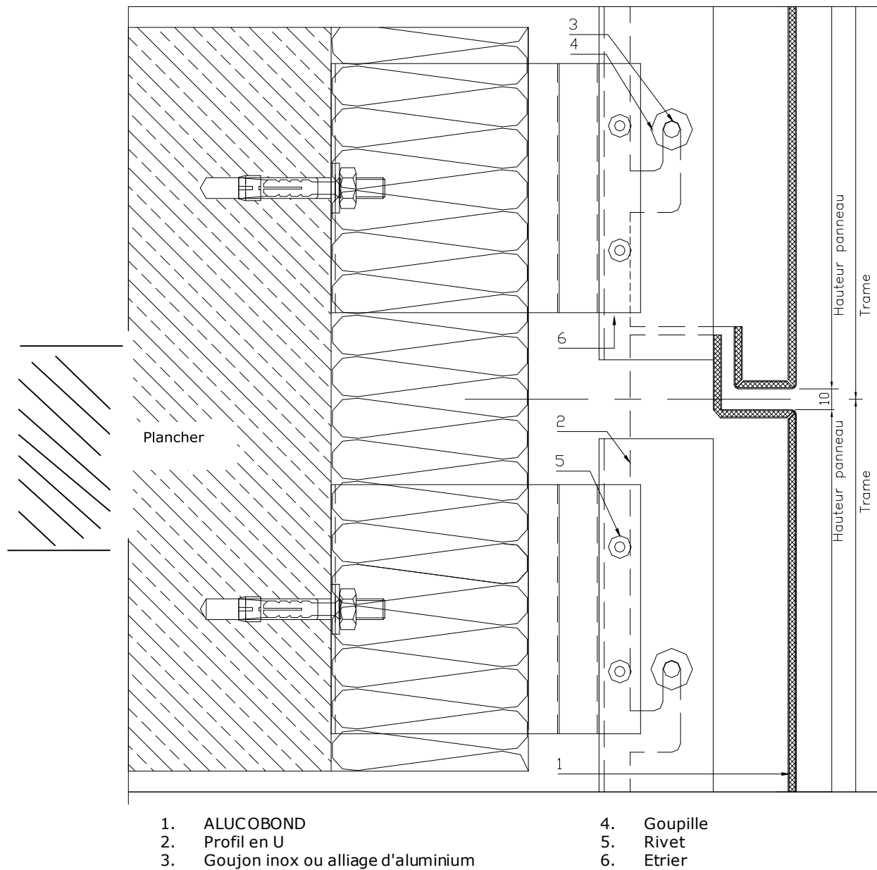
Figure A1 – Montage cassette - Coupe verticale au droit de chaque plancher
