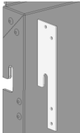
Figure 8 – Renfort d'encoche aux coins de la cassette avec une tôle d'angle en aluminium EN AW-5754 t = 2 \text{ mm} ou t = 3 \text{ mm} (cf. du Tableau 4 au Tableau 14 pour plus de précisions)
