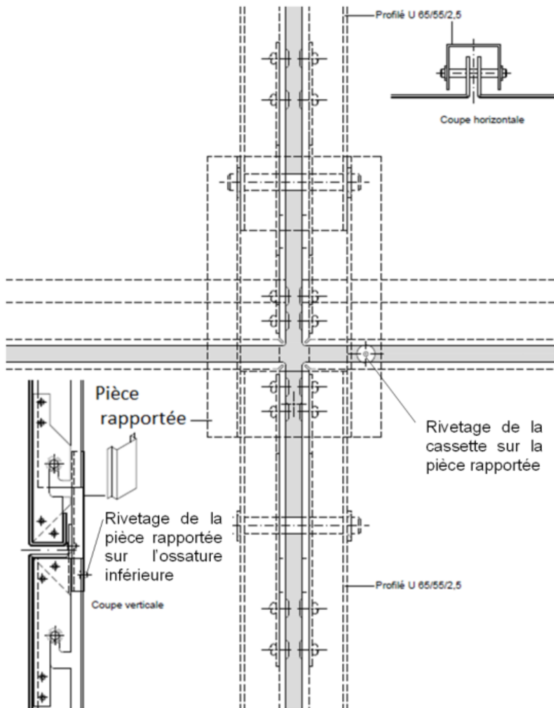
Figure 20 – Joint horizontal entre panneaux avec point fixe de cassette pour un système d'ossature en U (Elévation)
