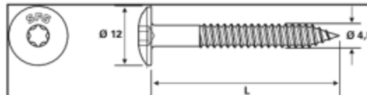
Figure 5 – Fixations des agrafes
