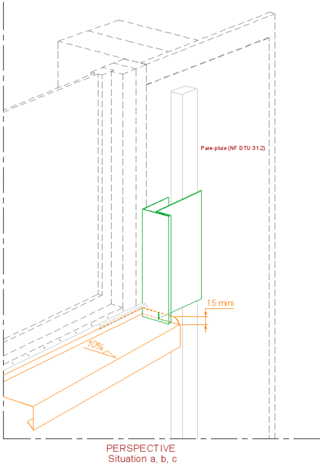
Figure 18 – Pose sur COB – Perspective – Dispositions particulières du traitement des baies (menuiserie en tunnel intérieur)
