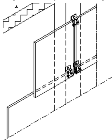
Figure 1 - Disposition des agrafes
