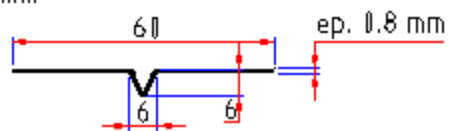
Profilé de jonction
