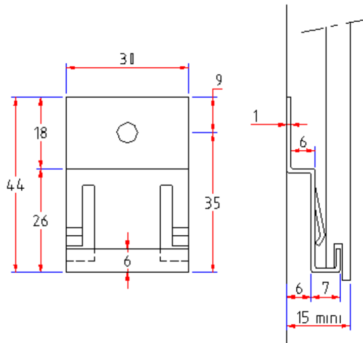
Figure 3 - Détail agrafe
