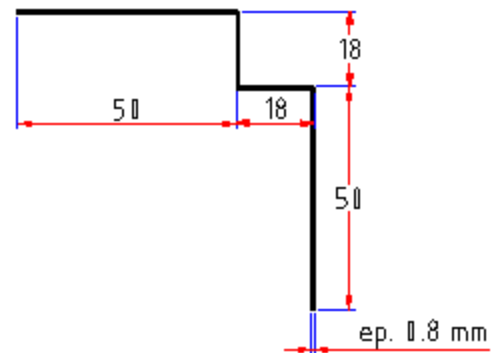
Profilé d'angle sortant croix
