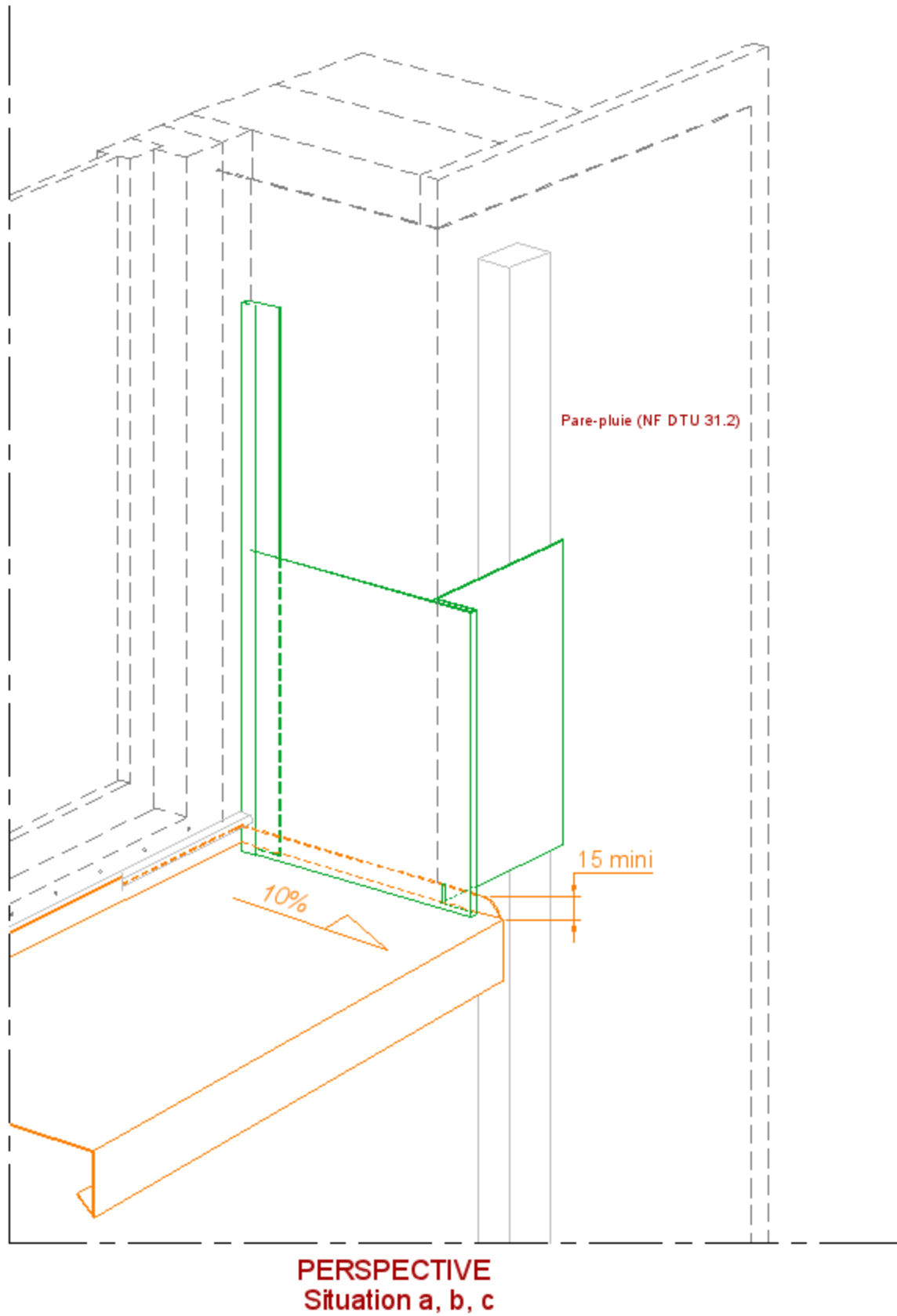
Figure 14 – Pose sur COB - Perspective – Dispositions particulières du traitement des baies (menuiserie en tunnel intérieur)
