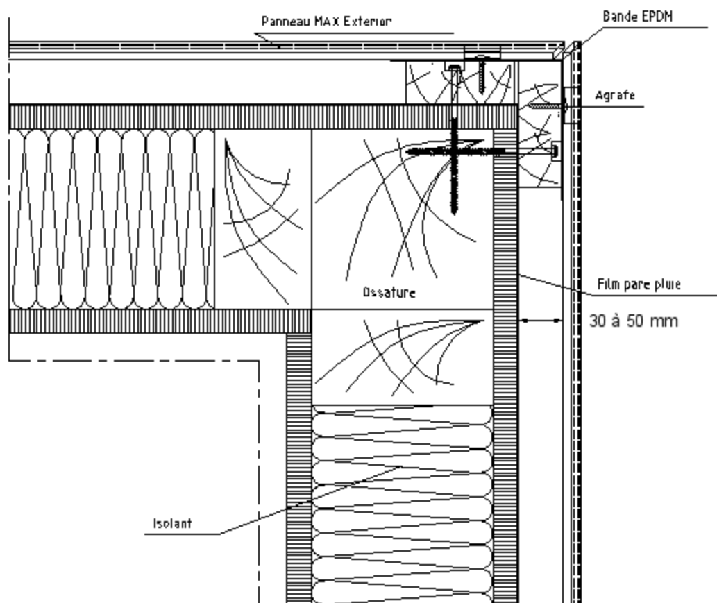
Figure 9 – Angle sortant sur COB jusqu'à 10 m
