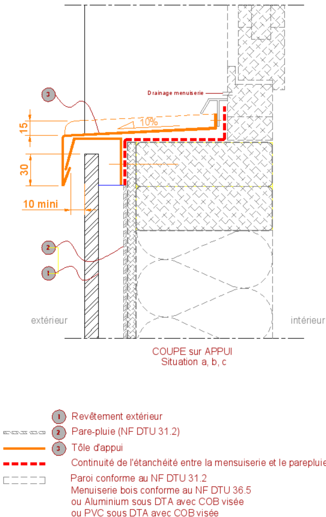
Figure 12 – Pose sur COB - Coupe sur appui de baie – Dispositions particulières du traitement des baies (menuiserie en tunnel intérieur)
