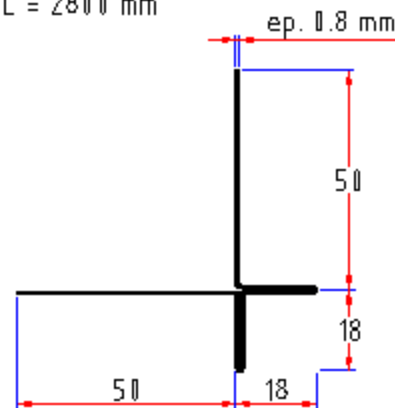
Profilé d'angle sortant croix
