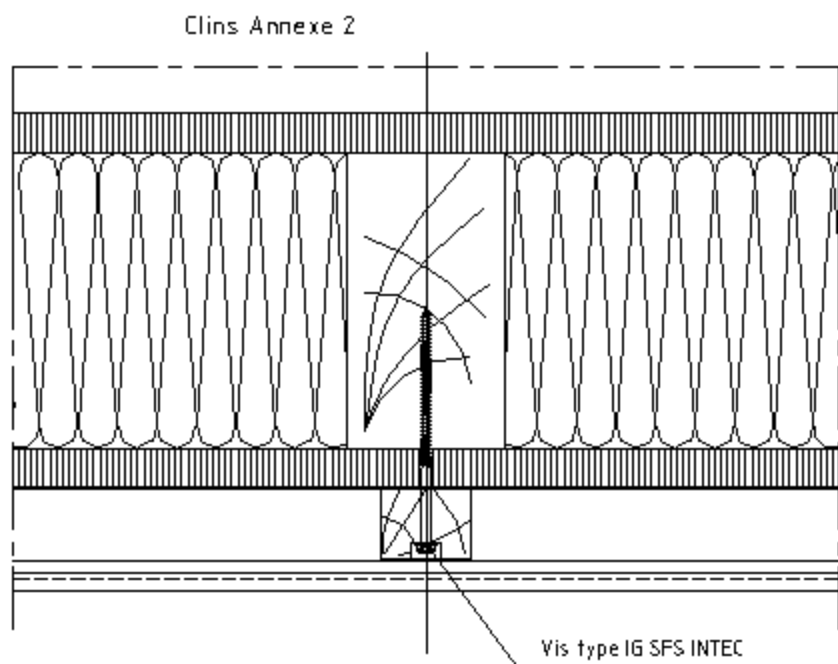
Figure A2 – Joint vertical intermédiaire – Pose sur COB
