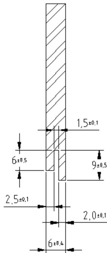
Figure 4 - Détail clin usinage
