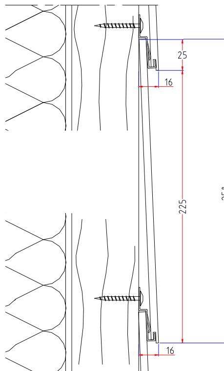
Figure 6 - Profils d'habillage
