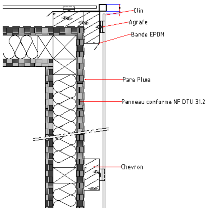
Figure 10 – Pose sur COB
