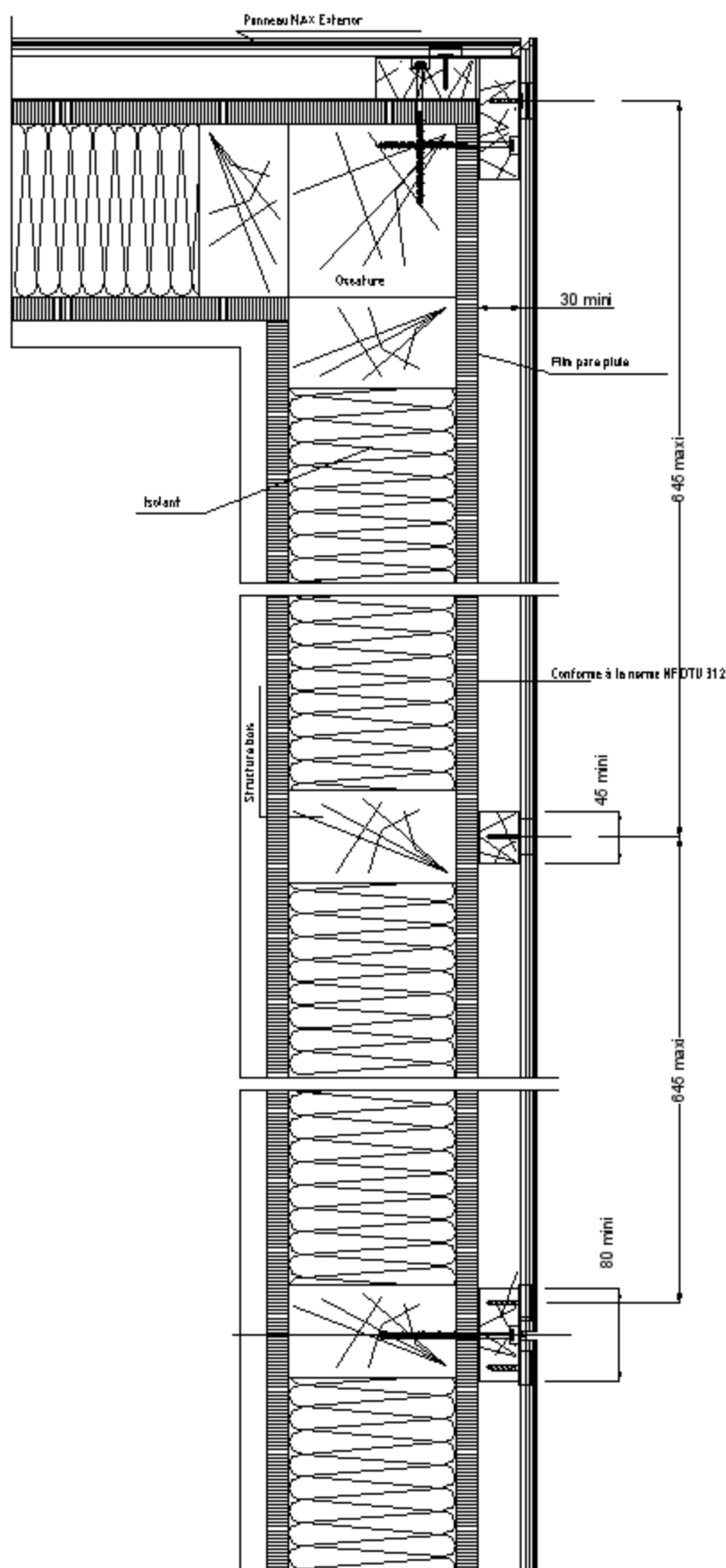
Figure 8 – Pose sur COB
