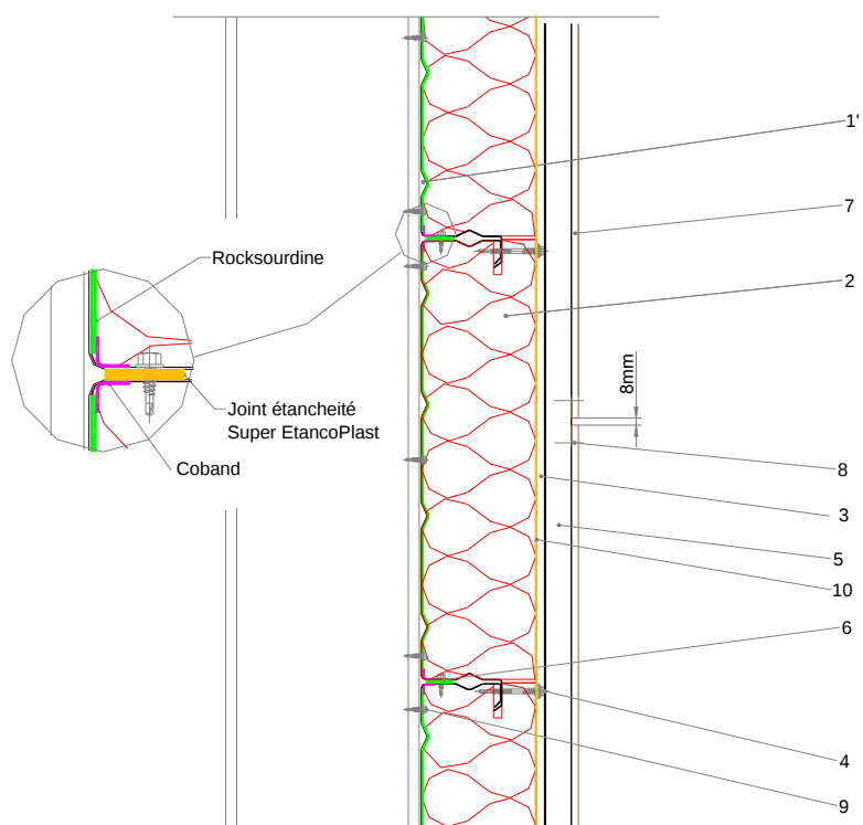
Figure 6 – Coupe verticale en partie courante (avec Rocksource sur plateaux perforés)
