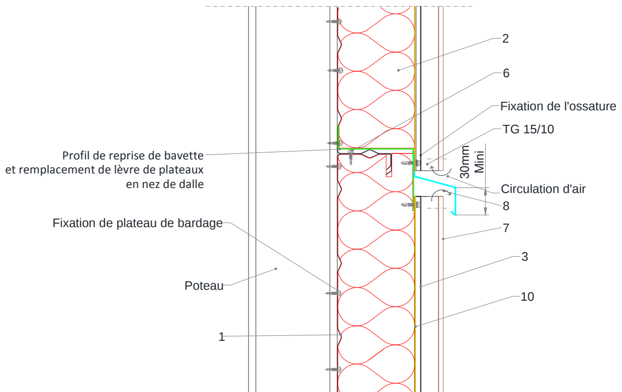
Figure 12 – Fractionnement de lame d'air – Coupe verticale
