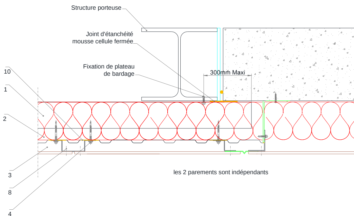
Figure 21 – Jonction sur maçonnerie
