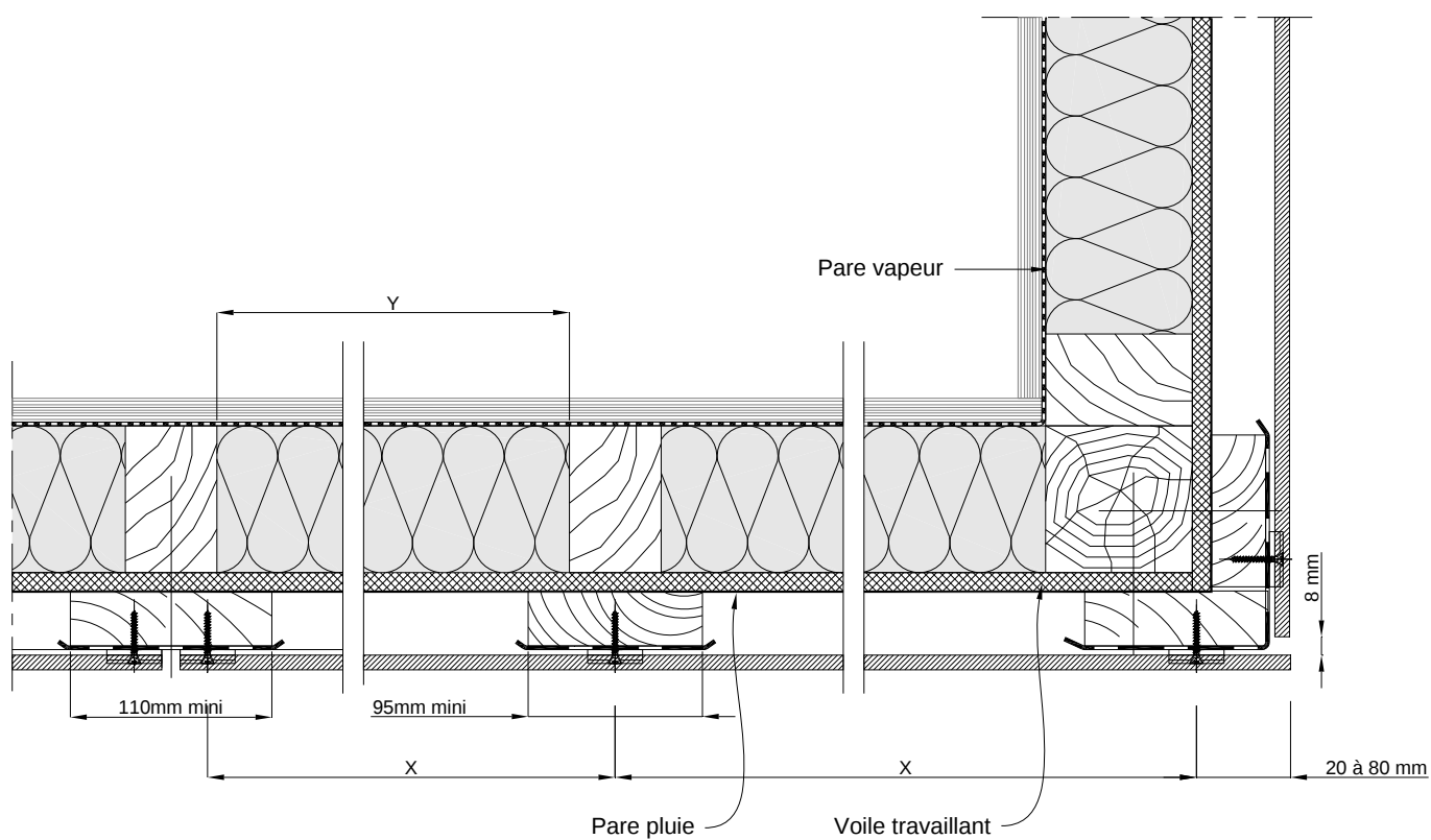
Figure 37 - Pose horizontale - Coupe horizontale sur COB/CLT
