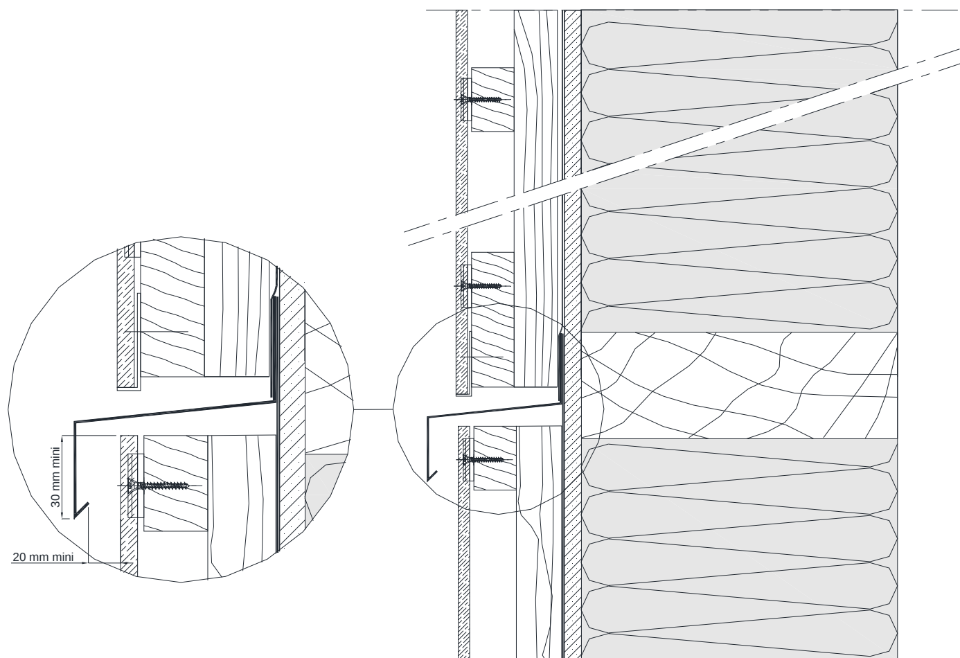
Figure 42 - Pose verticale - Recouplement du pare-pluie tous les 6m
