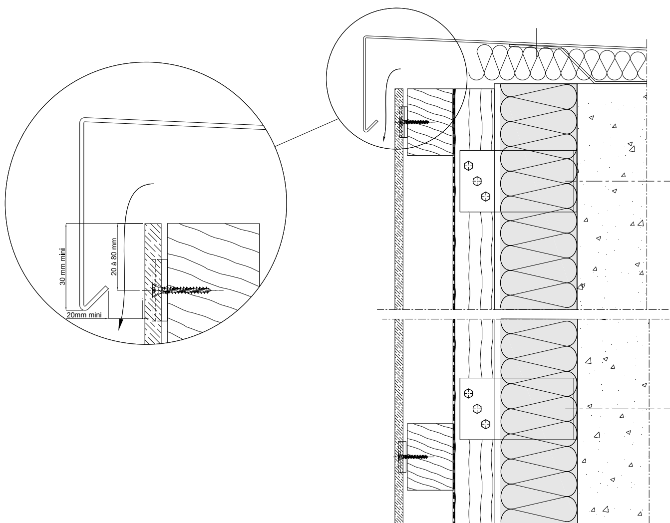
Figure 21 - Pose verticale - Arrêt sur acrotère
