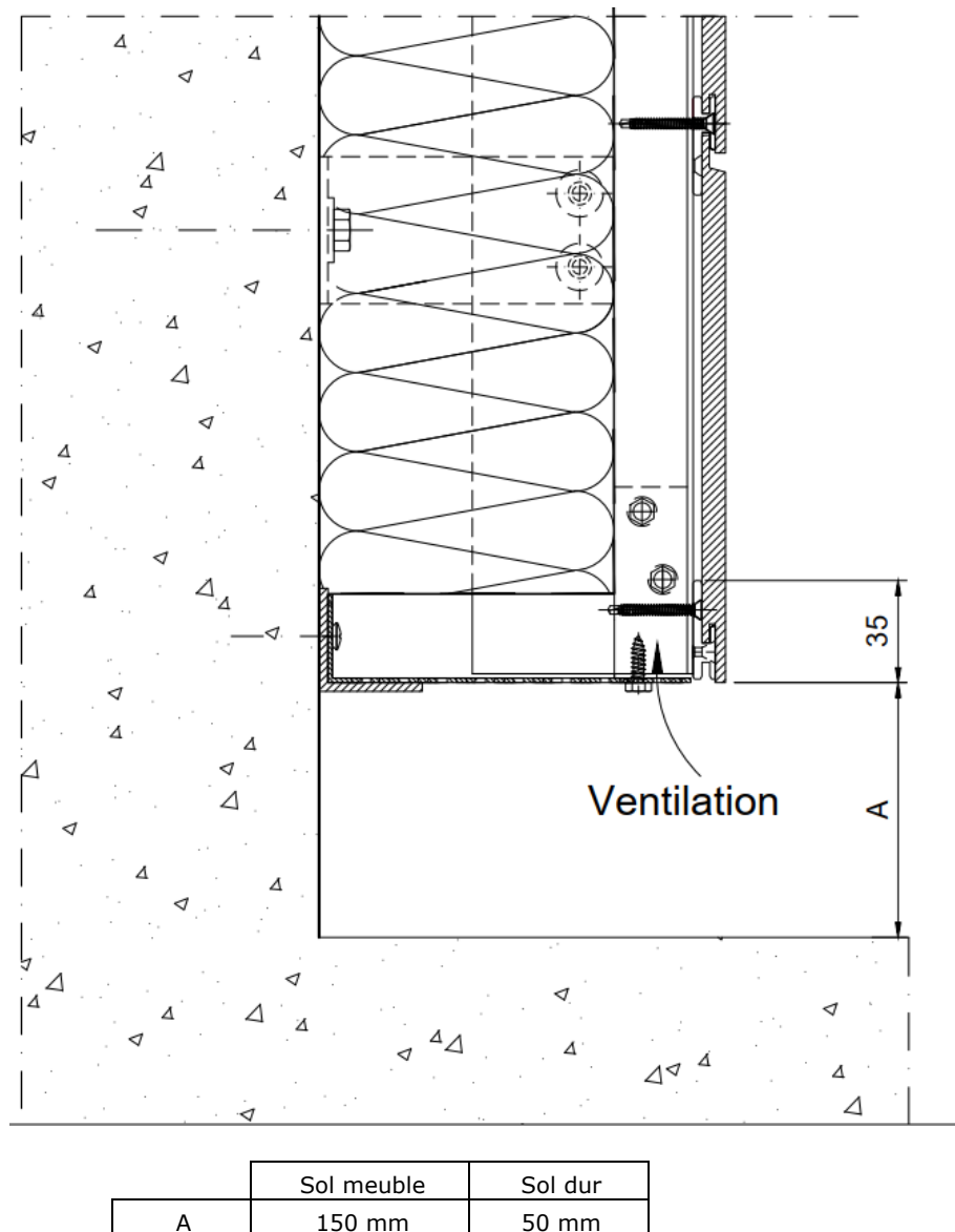
Figure 46 – Départ de bardage en pose horizontale sur ossature aluminium
