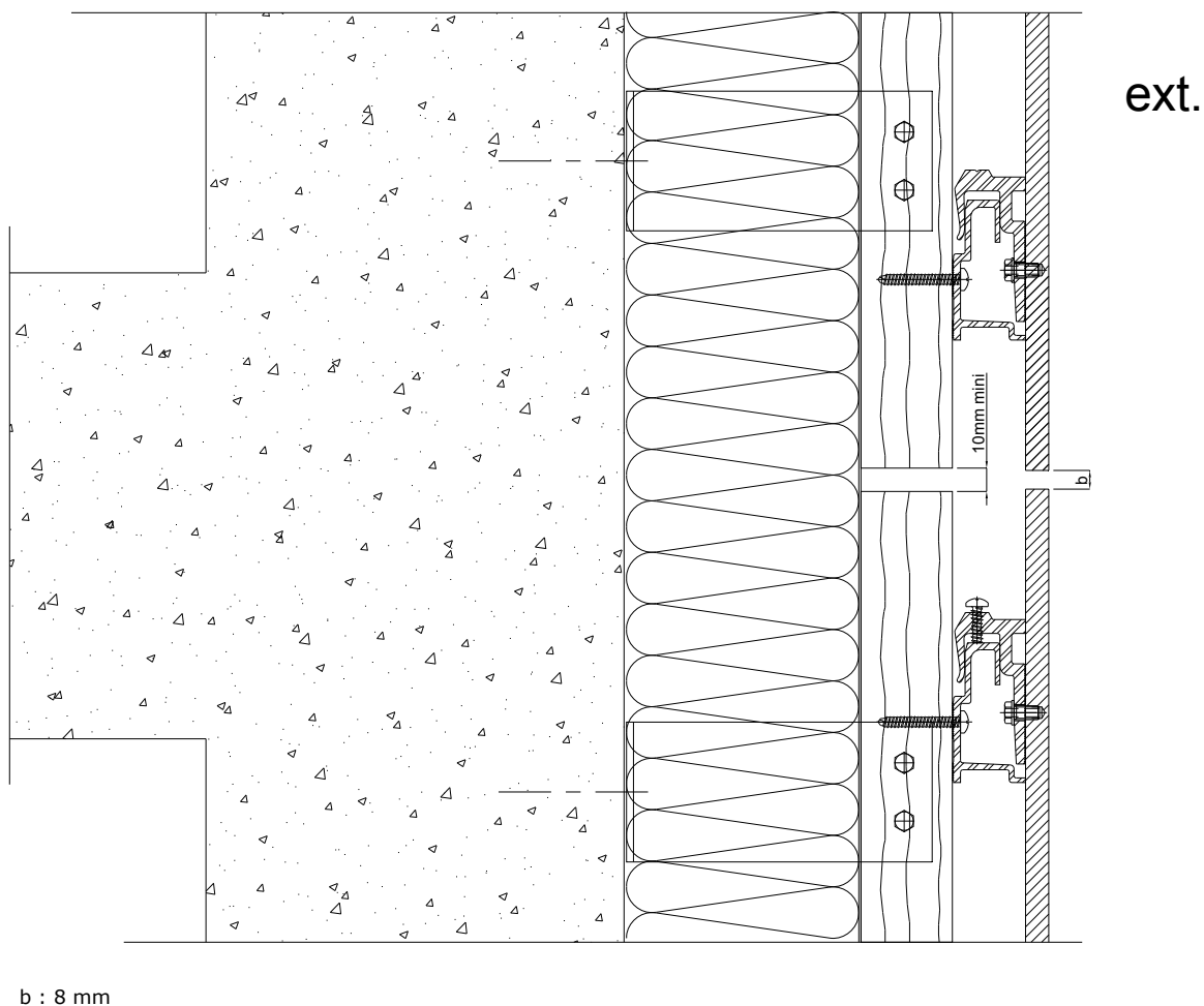
Figure A5 – Fractionnement au droit des planchers – ossature bois
