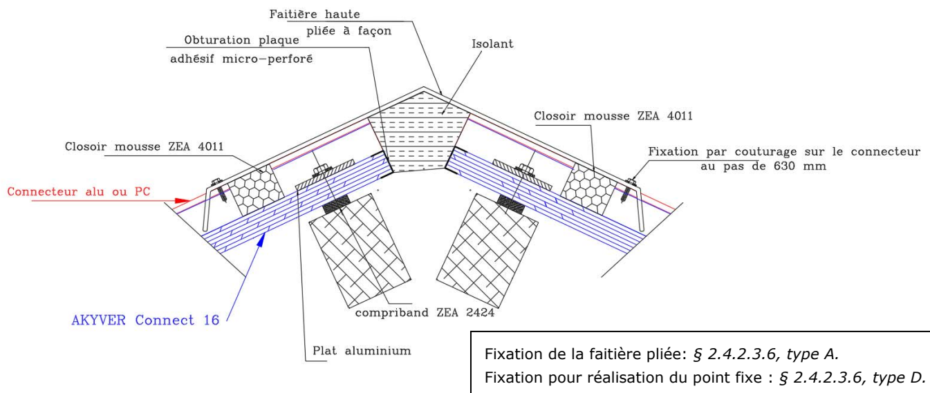
Figure 17 – Faîtage avec point fixe haut
