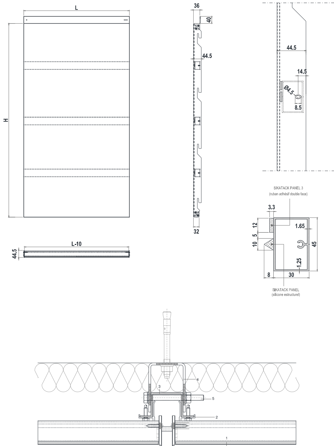
Figure 24bis – Exemple de disposition des raidisseurs horizontaux collés
