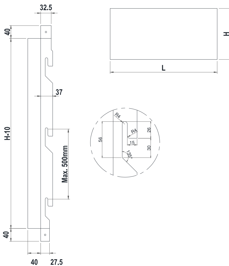
Figure 4a – Raidisseur vertical collé
