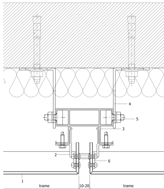
Figure 2bis – Système avec profilé LC-2 – Vue horizontale
