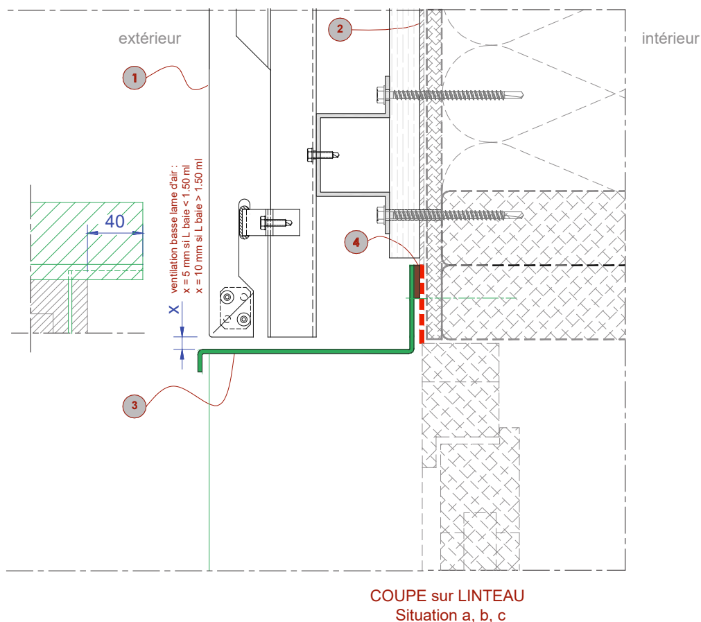
Figure 20 – Pose sur COB – Coupe sur linteau de baie, applicable sur COB (cf. § 2.11.2) ou sur CLT (cf. § 2.11.3) Dispositions particulières du traitement des baies (Menuiserie en tunnel au nu extérieur)
