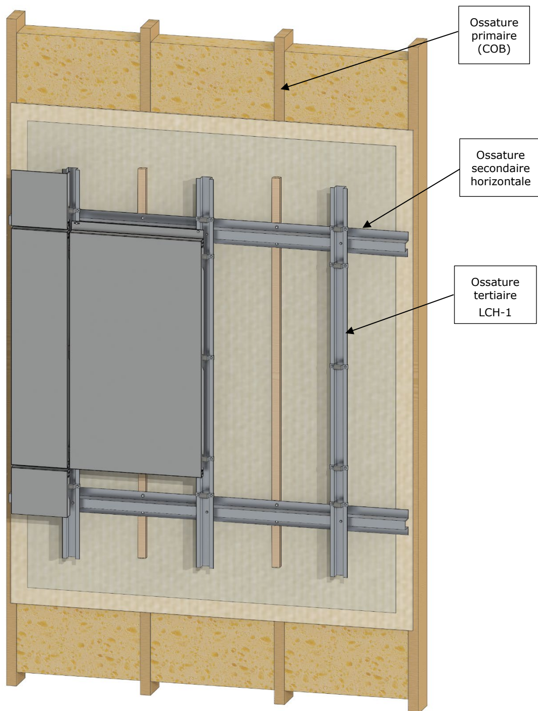
Figure 1 – Principe de mise en œuvre du system LARSON cassette sur COB
