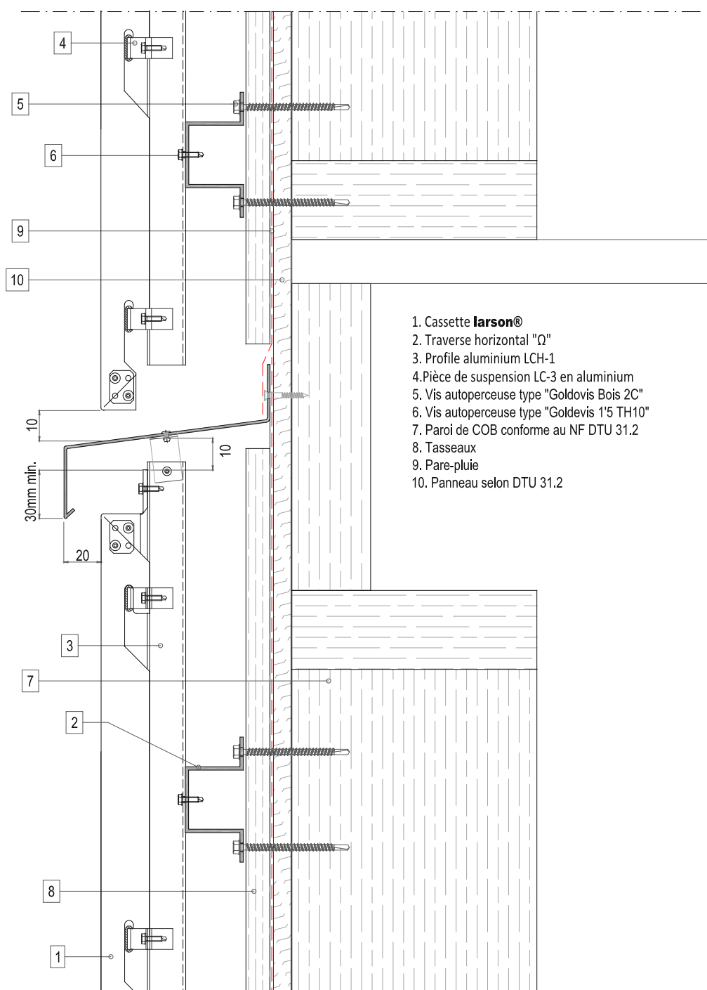
Figure 15– Fractionnement de la lame d'air et recoupement du pare-pluie
