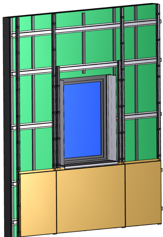
Etape 6 – Pose des cassettes larson® en allège.
