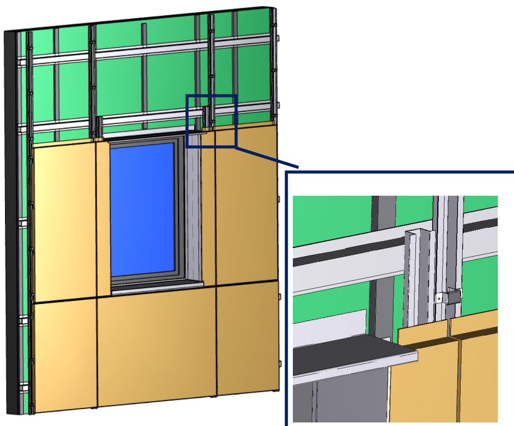
Etape 8 – Pose de l'habillage de linteau.
