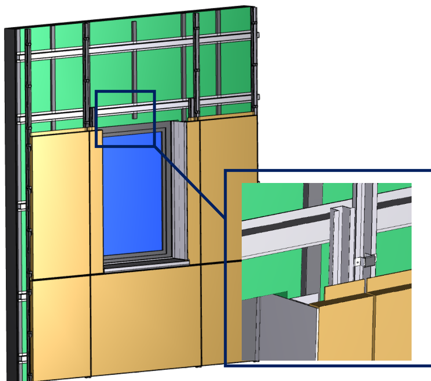
Etape 7 – Pose des cassettes larson® de part et d'autre de la menuiserie et grugeage du pli haut de cassette pour passage de l'habillage de linteau.
