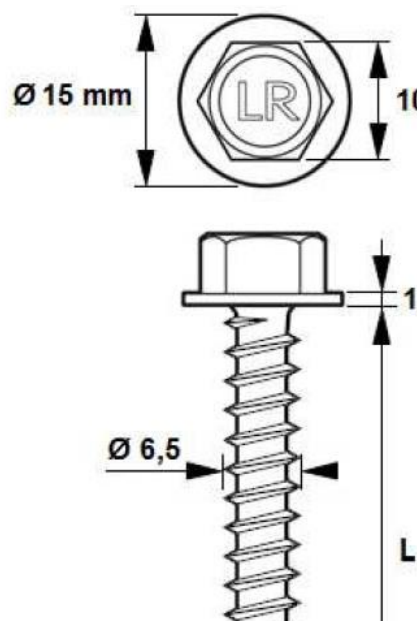
Figure 2c – Vis de fixation sur COB - Goldvis bois TH 10 de la Société Etanco
