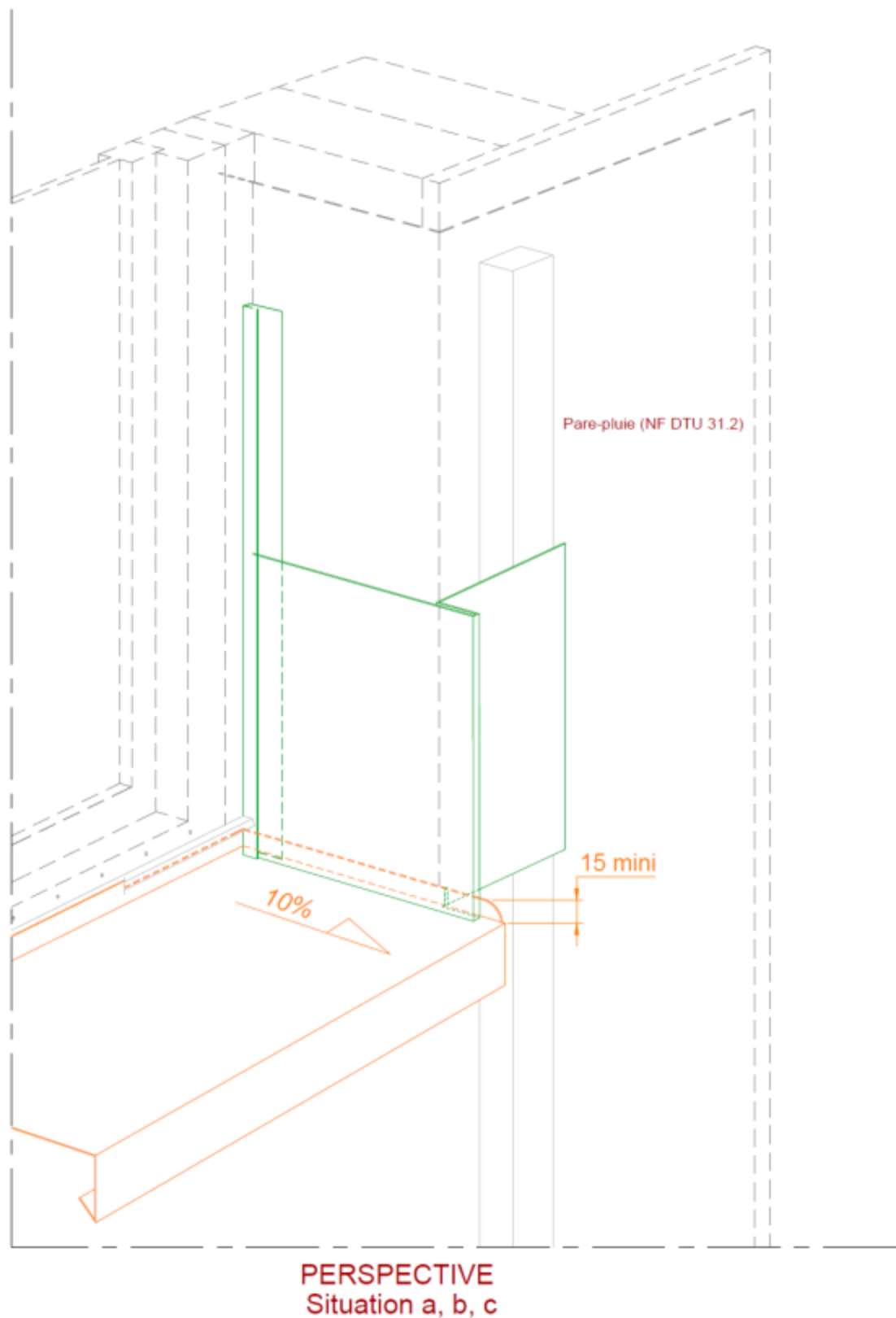
Figure 16 --Perspective Dispositions particulières du traitement des baies (Menuiserie en tunnel intérieur) Hauteurs de COB \leq 18 m pour les situations a, b et c et < 10 m en situation d
