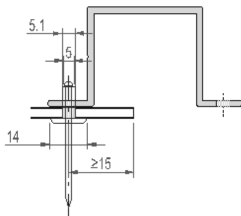
Rivet et fixation (point fixe)
