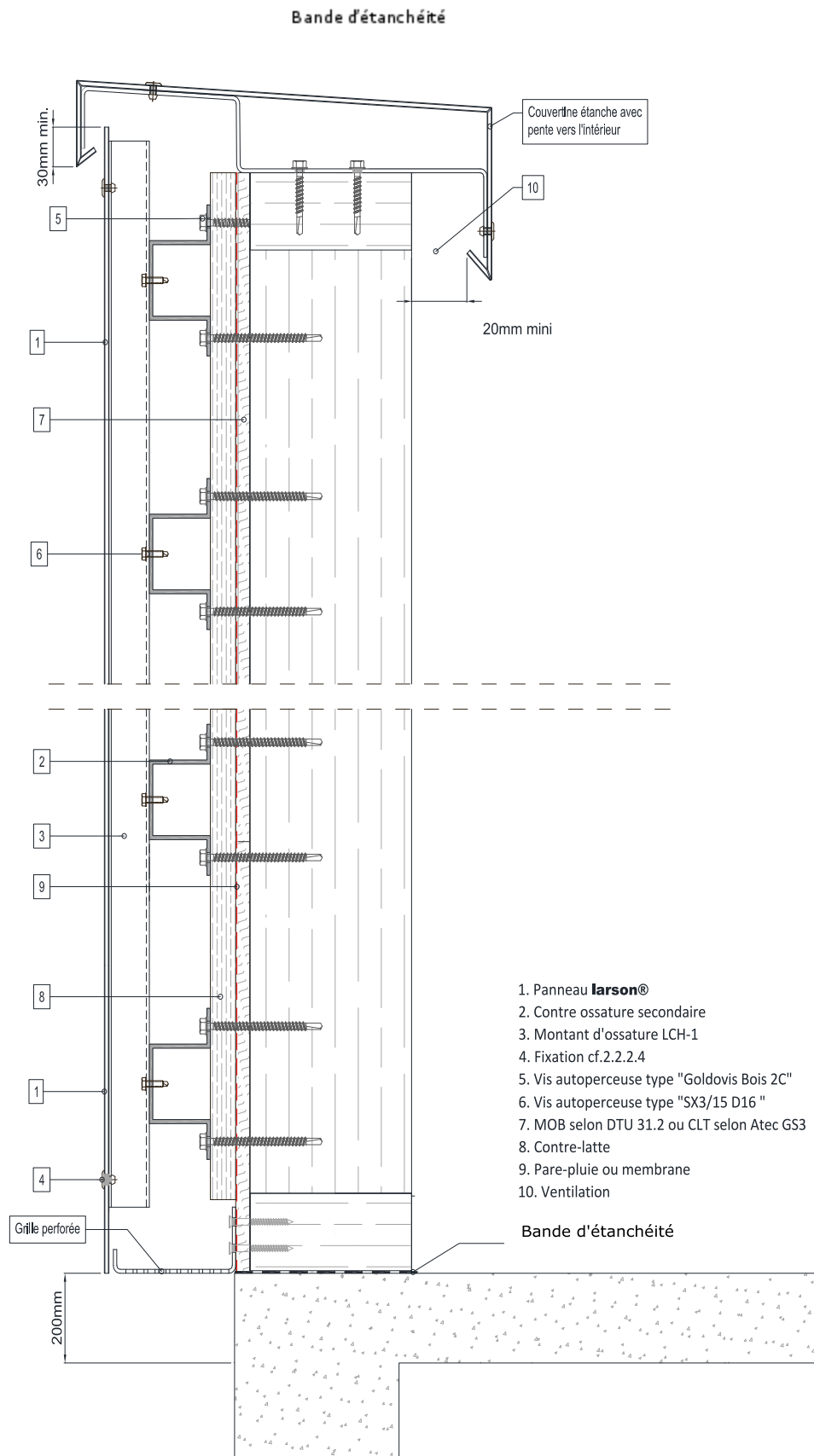
Figure 7 – Coupe verticale de principe sur COB
