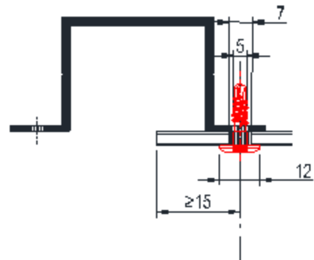
Vis de fixation (point coulissant)
