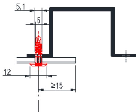
Vis de fixation (point fixe)
