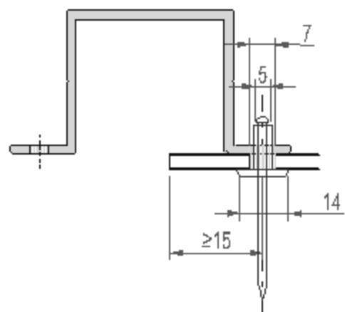
Rivet et fixation (point coulissant)
