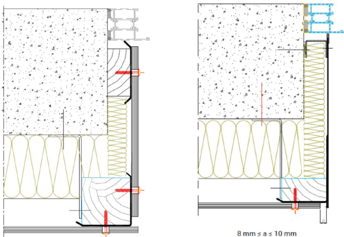
Figure 6 - Traitement des liaisons au niveau des baies : En tableau
