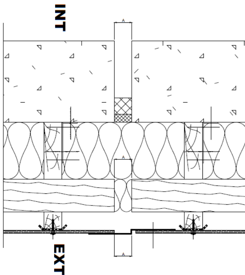
Figure 14– Traitement sur BA en multi réseau - Joint de dilatation – coupe horizontale
