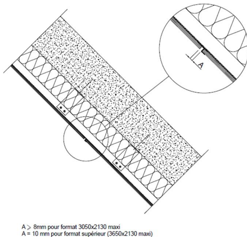
Figure 7 - Traitement sur paroi inclinée
