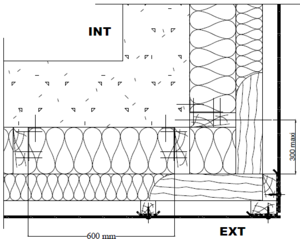
Figure 10- Traitement sur BA en multi réseau - Coupe horizontale angle rentrant
