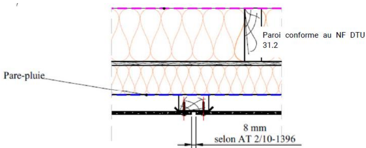
Figure 19 - Traitement sur COB/CLT avec complément d'isolation par l'extérieur - Coupe horizontale en paroi courante
