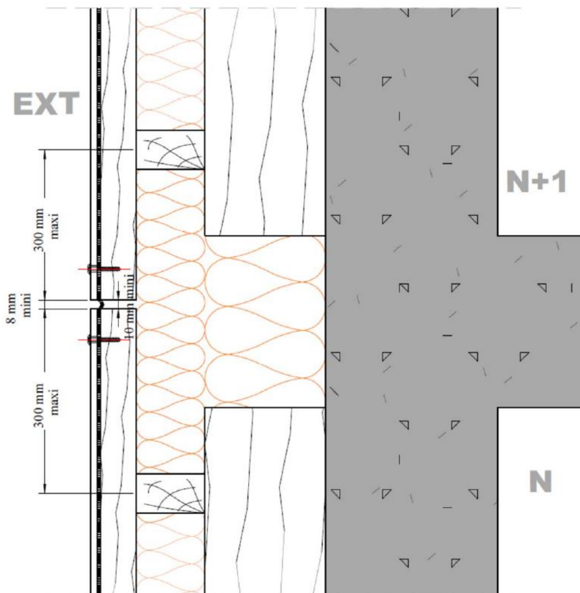
Figure 15– Réseaux croisés sur BA - Fractionnement de l'ossature au droit de chaque plancher
