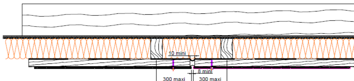
Figure 22- Traitement sur COB/CLT avec complément d'isolation par l'extérieur - Pose en sous-face sur COB
