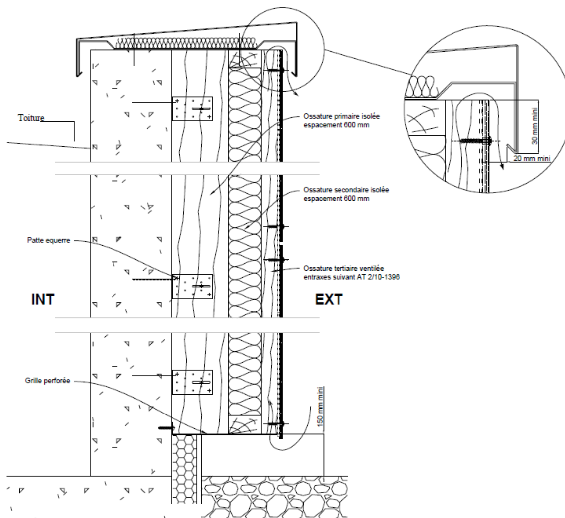
Figure 9 - Traitement sur BA en multi réseau sur béton - Coupe verticale générale
