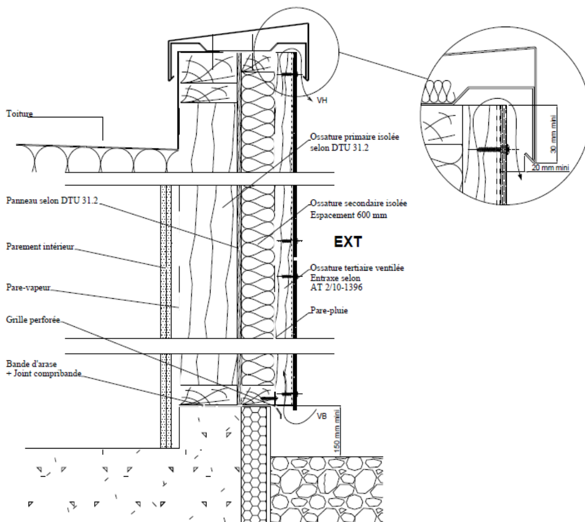
Figure 16- Traitement sur COB/CLT avec complément d'isolation par l'extérieur - Coupe verticale générale
