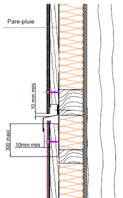
Figure 21- Traitement sur COB/CLT avec complément d'isolation par l'extérieur - Recouplement du pare-pluie tous les 6 m avec le système multi-réseaux
