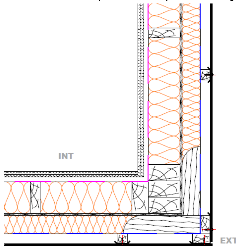
Figure 18- Traitement sur COB/CLT avec complément d'isolation par l'extérieur - Angle sortant
