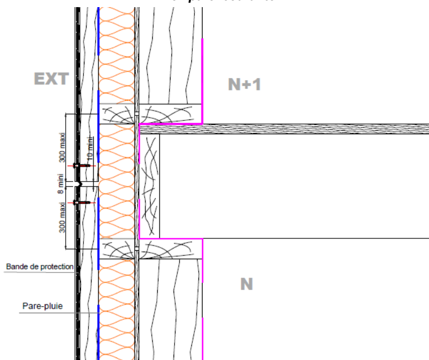
Figure 20- Traitement sur COB/CLT avec complément d'isolation par l'extérieur - Fractionnement de l'ossature au droit de chaque plancher
