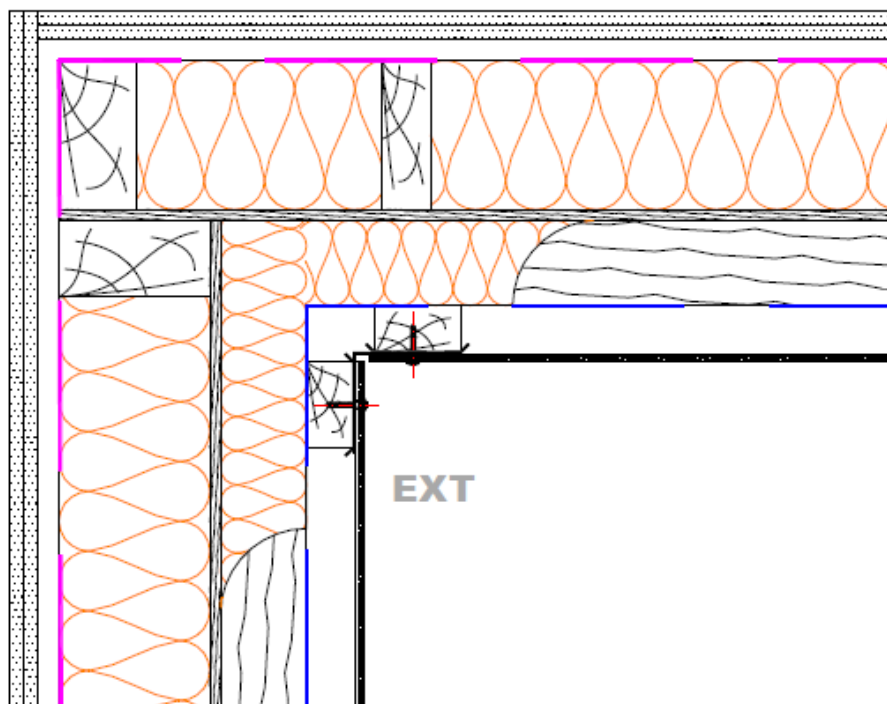
Figure 17 - Traitement sur COB/CLT avec complément d'isolation par l'extérieur - Angle rentrant
