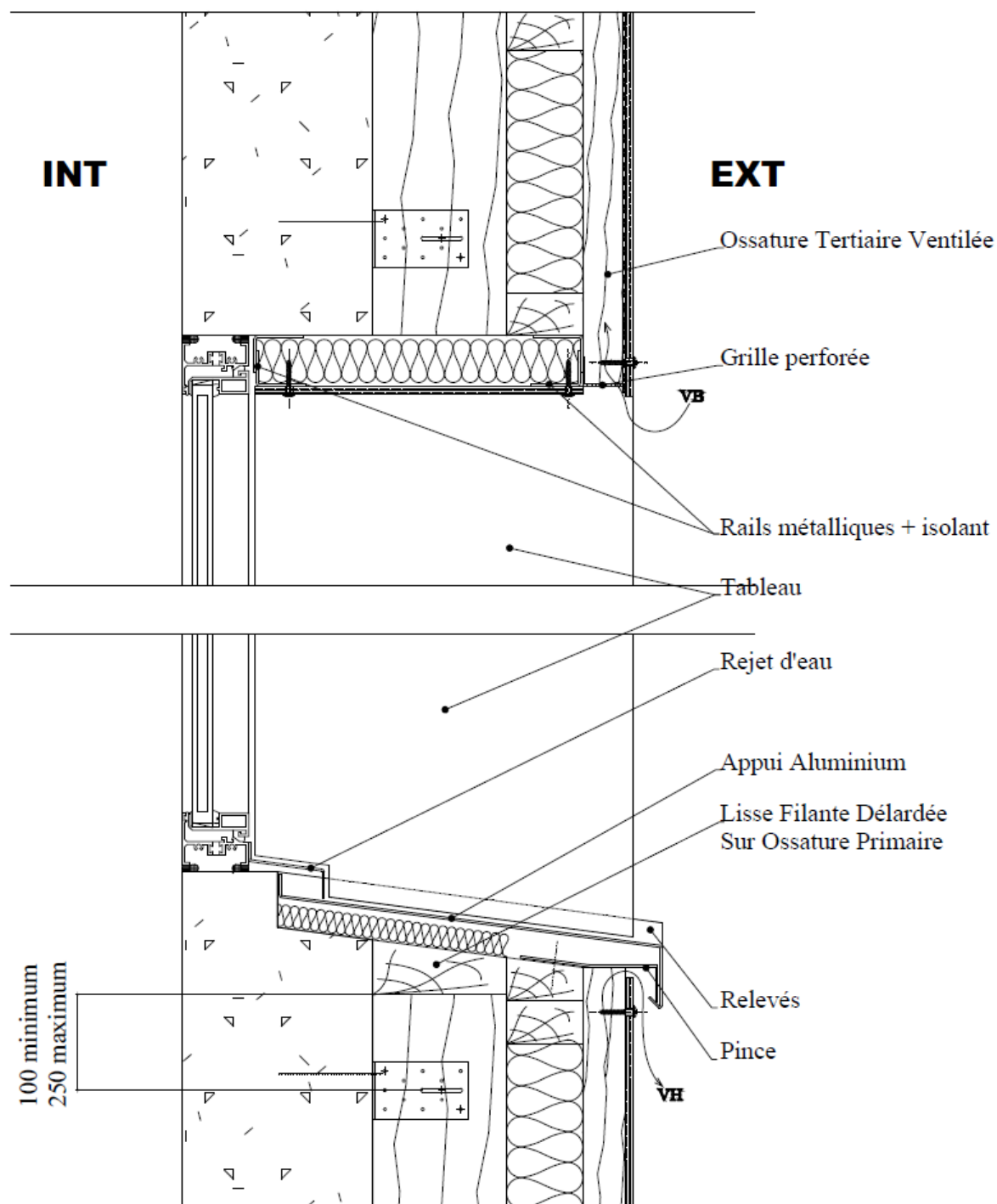
Figure 12– Traitement sur BA en multi réseau - Coupe verticale sur voussure et appui de menuiserie
