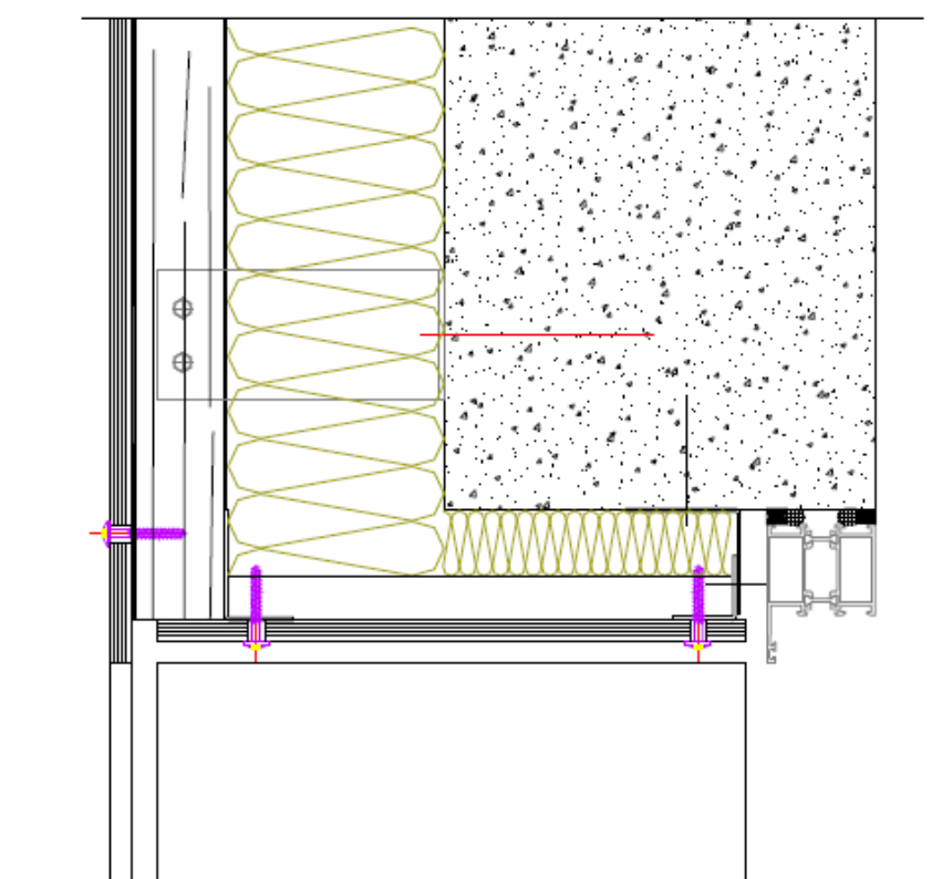
Figure 5 - Traitement des liaisons au niveau des baies : En linteau
