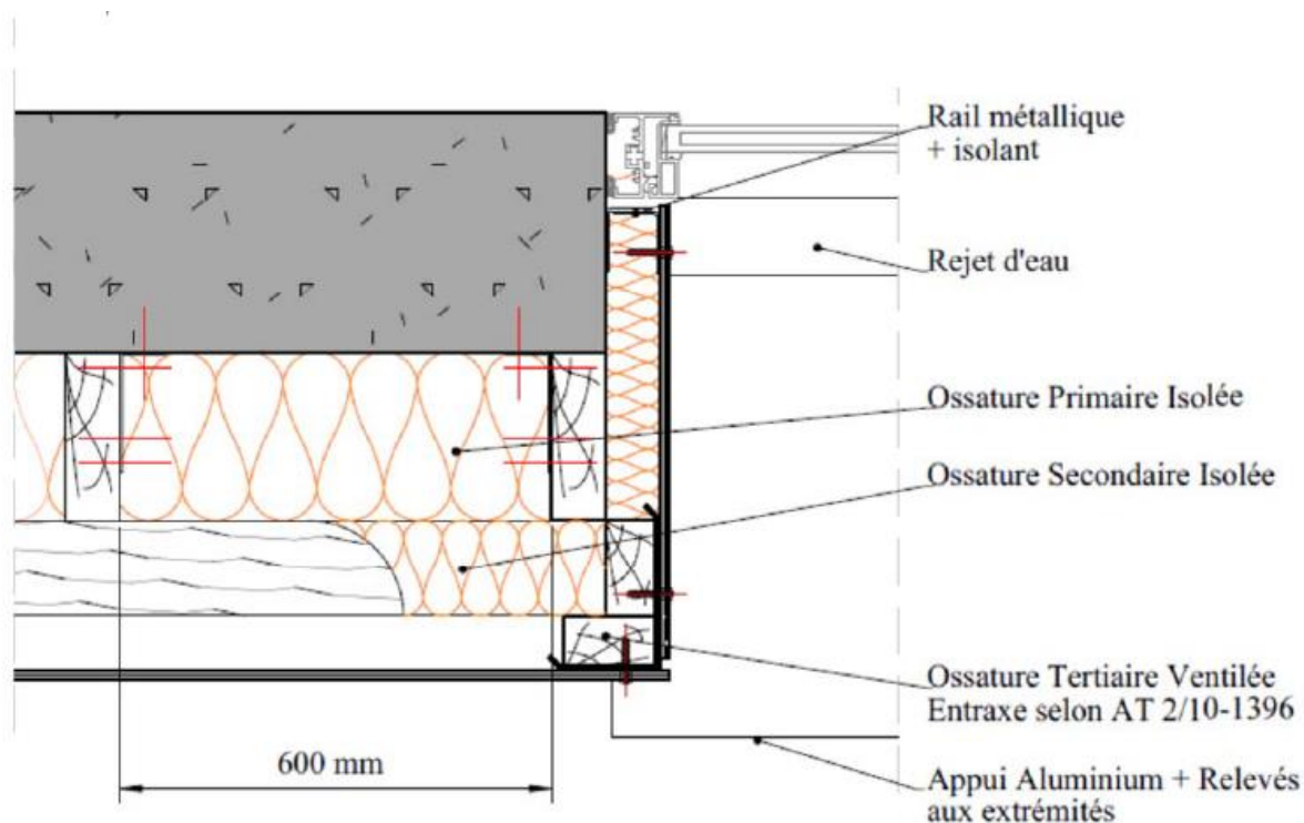
Figure 13– Traitement sur BA en multi réseau -Coupe sur tableau
