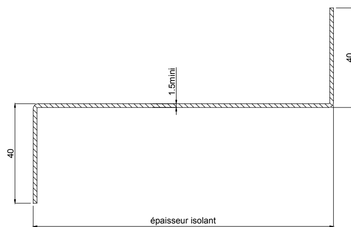
Figure 6 - Profil de reprise de bavette et de remplacement de lèvre de plateau
