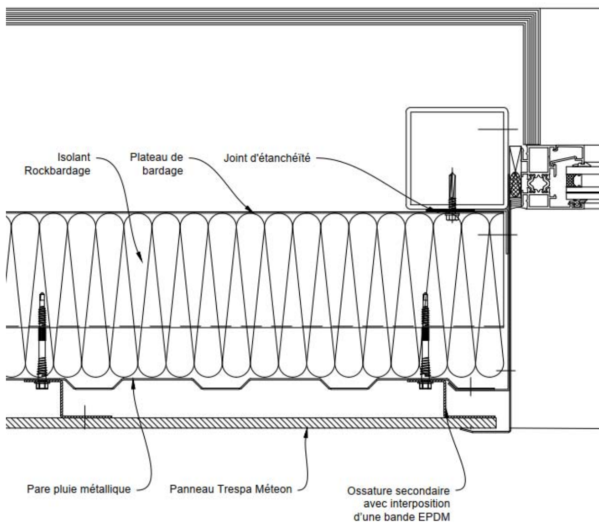
Figure 20 - Coupe sur tableau
