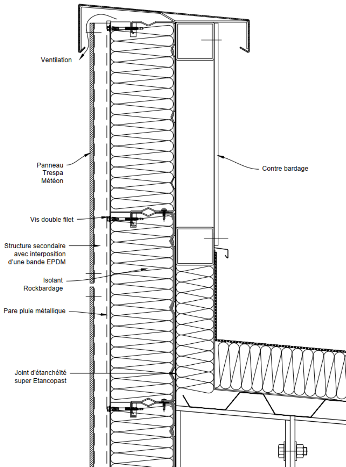
Figure 15 - Coupe verticale sur acrotère
